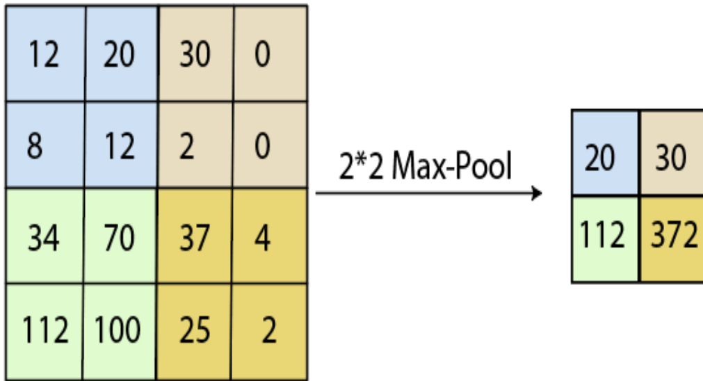
Fig 6 : Max Pooling(a)
